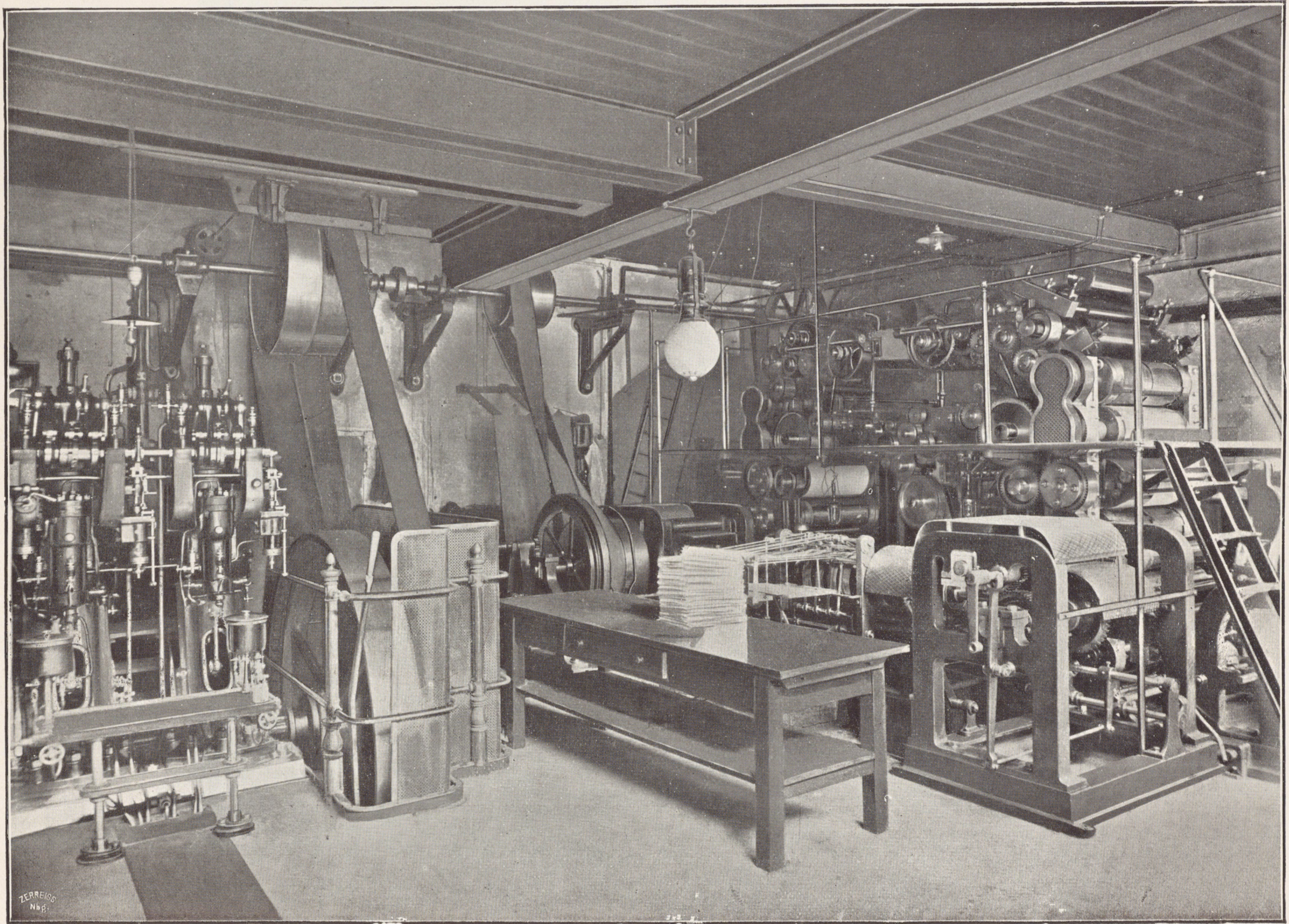
Nürnberg Maschinensaal (Diesel-Motor und Zwillings-Rotationsmaschine).
